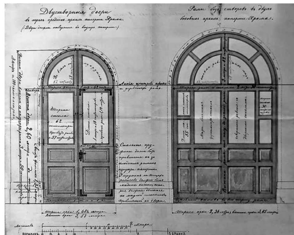
Чертеж дверей паперти Троицкого собора.
