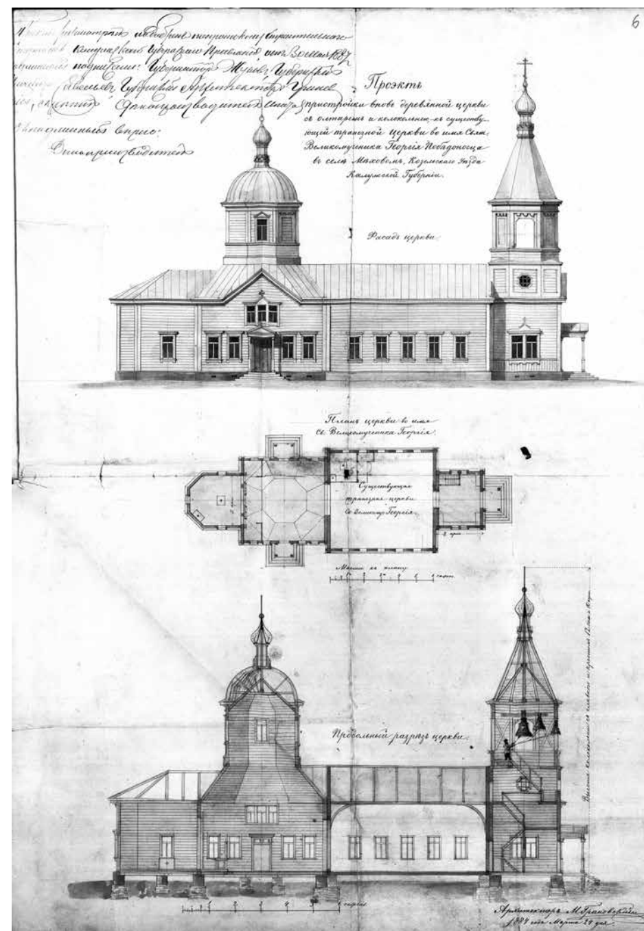
М.Ф. Грановский. Проект пристройки деревянной церкви с алтарем и колокольнею к существующей трапезной церкви во имя Свят. Великомученика Георгия Победоносца в с. Меховом Козельского уезда Калужской губернии. 1884 г. ГАКО.
