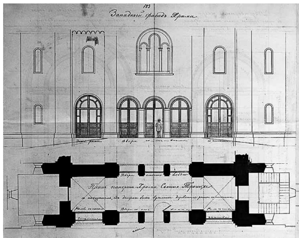
Чертеж западного фасада и план паперти Троицкого собора.
